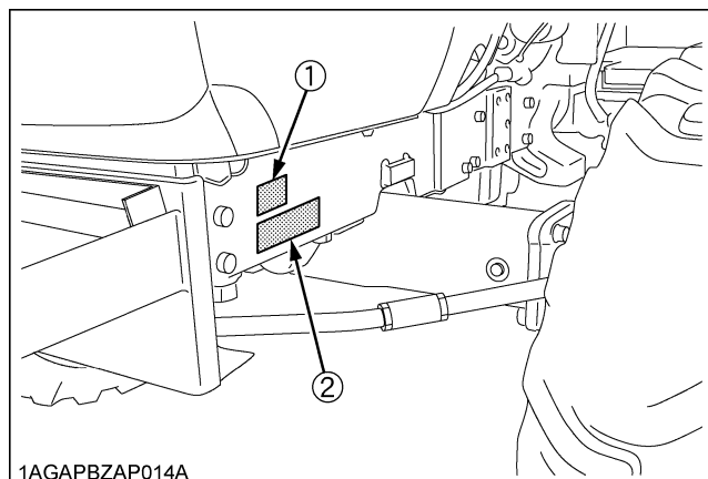
(1) Biển nhận dạng máy kéo (2) Số seri máy kéo
